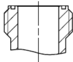
E NPTF Aussengewinde
