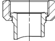
B Rotalockanschluss Innengewinde
