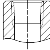
C NPTF Innengewinde
